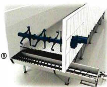
用於有機物進料接收的 KEITH 自動卸料地板
