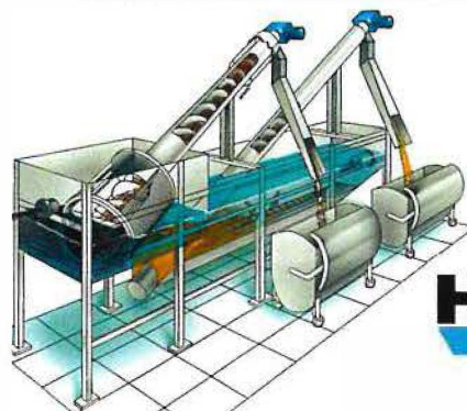
用於有機物 (漿料) 除砂的 HUBER 沉砂清洗系統
